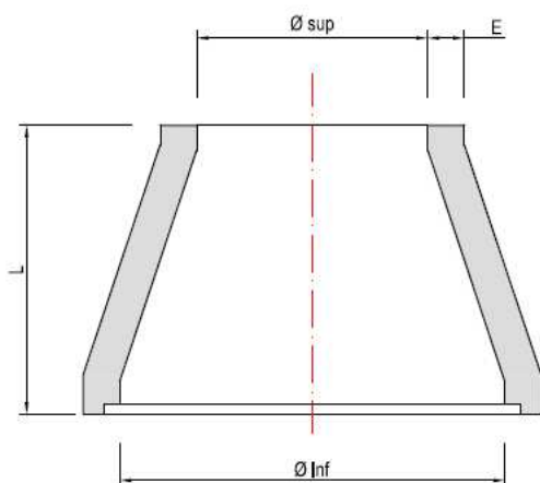
SECCION TIPO
